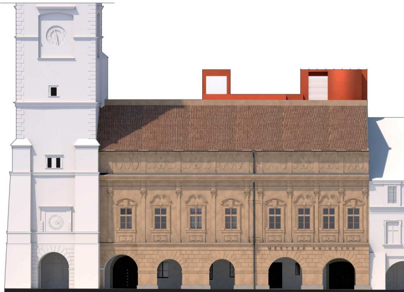
POHLED VÝCHODNÍ 0 5 10 m M 1:100
